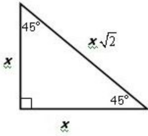
45-45-90 Triangle:
